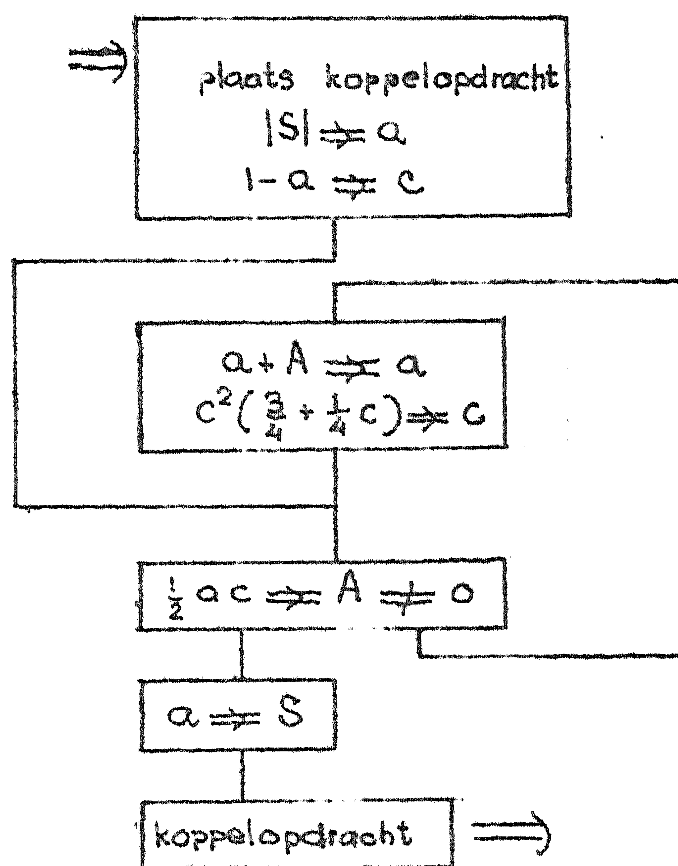
fig.3 |S|^{\frac{1}{2}} \neq S ; (repetitief)
