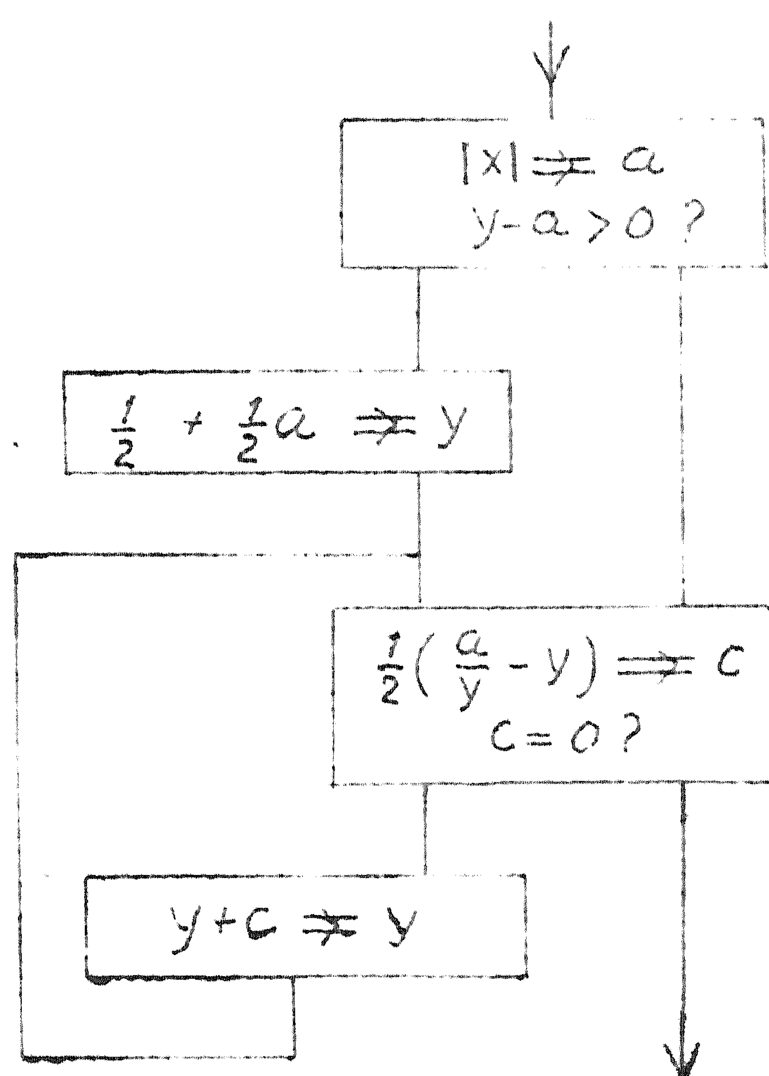
fig. 8 Blokschema |x|^{\frac{1}{2}} \Rightarrow y .
