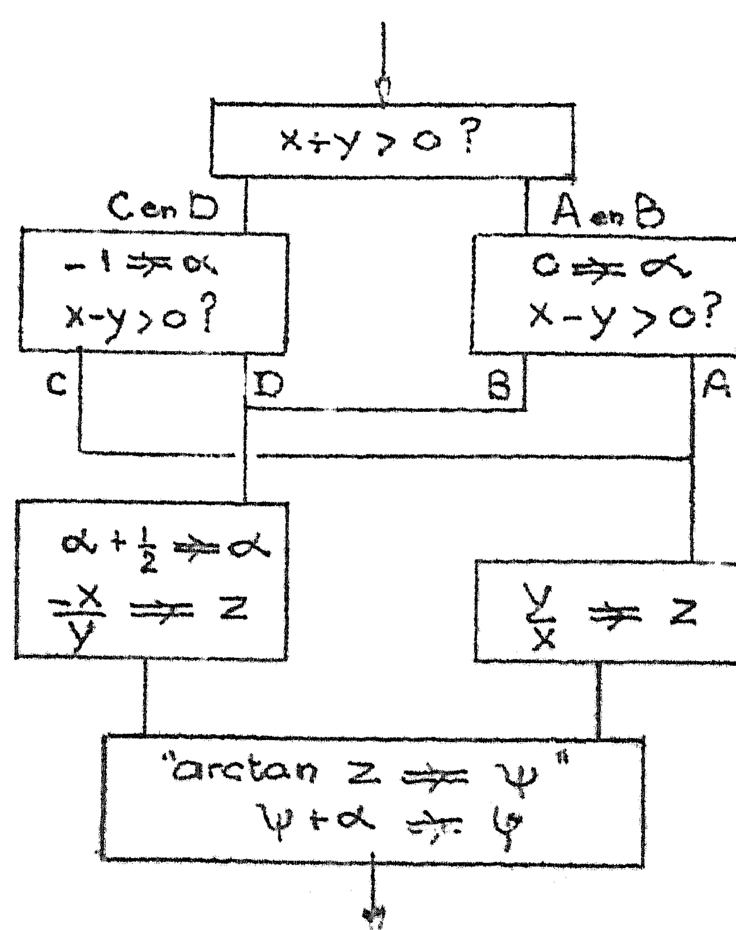
fig.4 Het "grove" blokschema: \arctan \frac{y}{x} \approx \varphi
